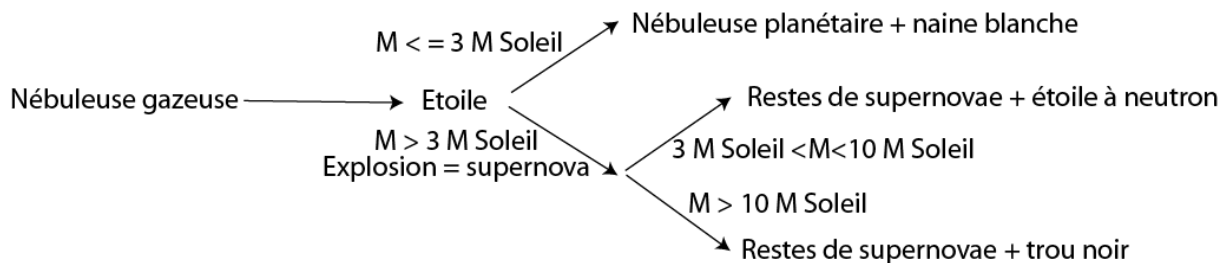
Figure 2 : Schéma de l'évolution des étoiles et des objets formés au cours de cette évolution
