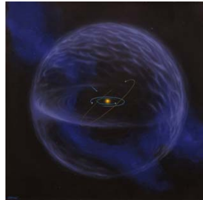
Photo 3 : le nuage d'Oort
