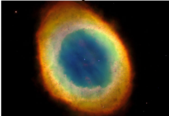
Photo 8 : nébuleuse planétaire
