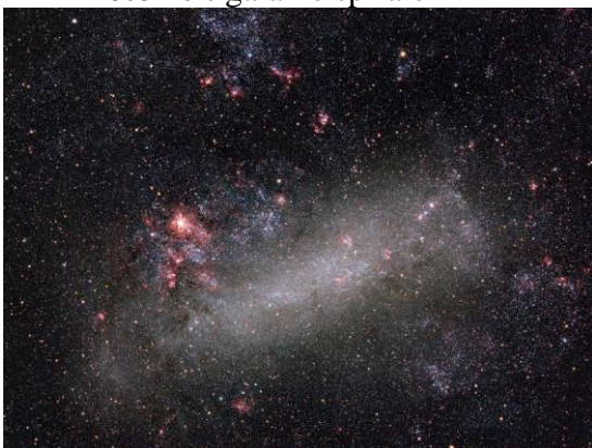
Photo 12 : galaxie irrégulière
