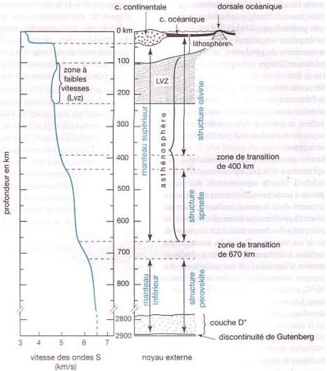
Figure 2 : Détails de la structure interne de la Terre selon les propriétés physiques. A gauche : variation des vitesses des ondes sismiques transversales (S). (D'après Brahic et al., 1999, Sciences de la Terre et de l'Univers)
