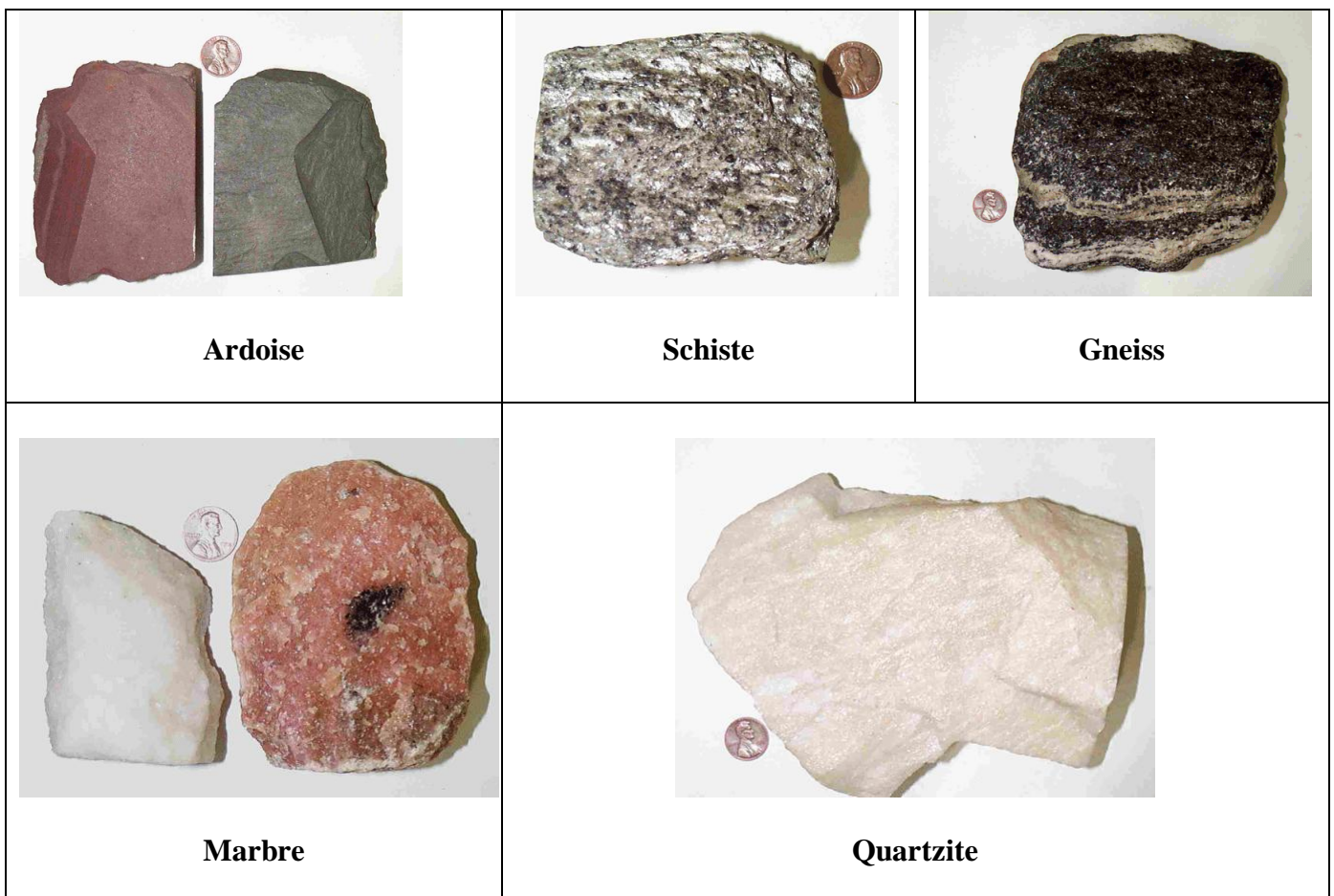
Figure 5 : Principales roches métamorphiques
