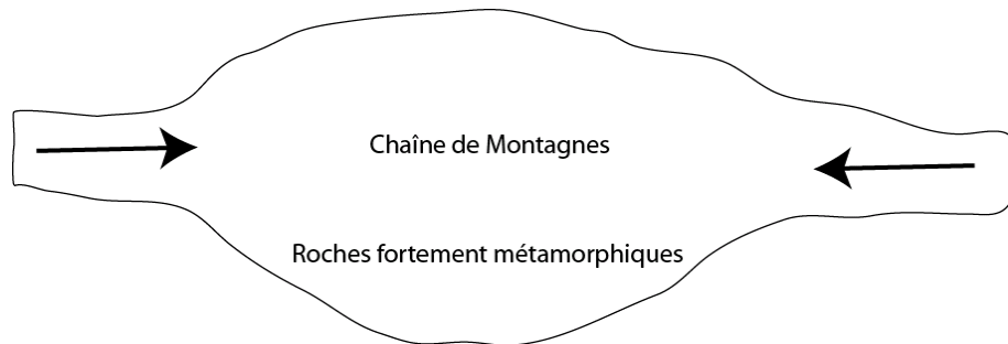
Figure 4 : le métamorphisme régional se produit au cœur des chaînes de Montagnes
