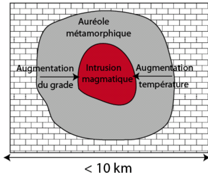
Figure 3 : métamorphisme de contact
